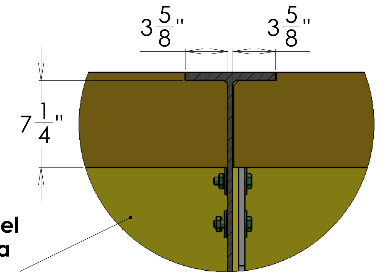
DETALLE L ESCALA 1:5
