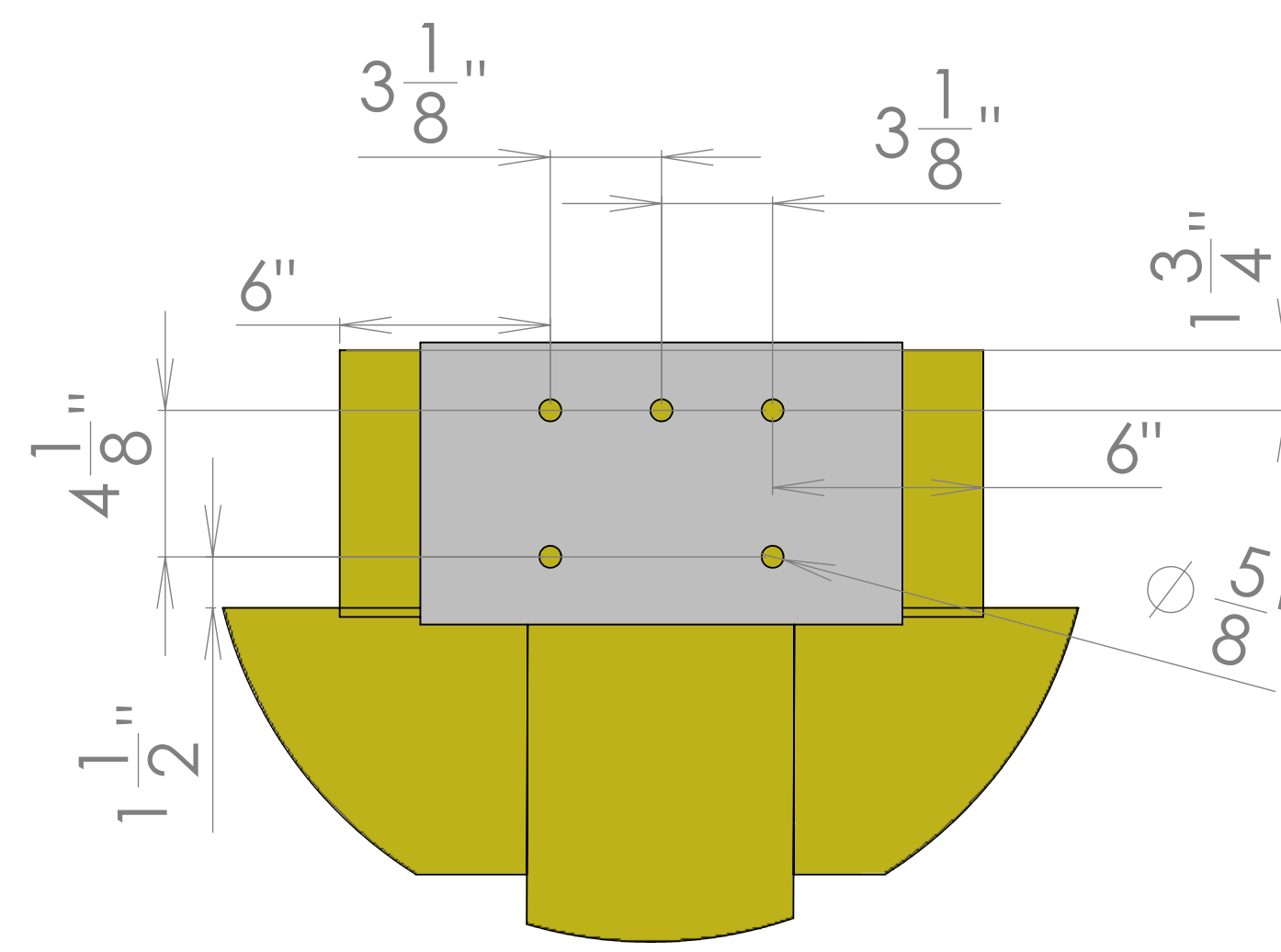
DETALLE C ESCALA 1:5
