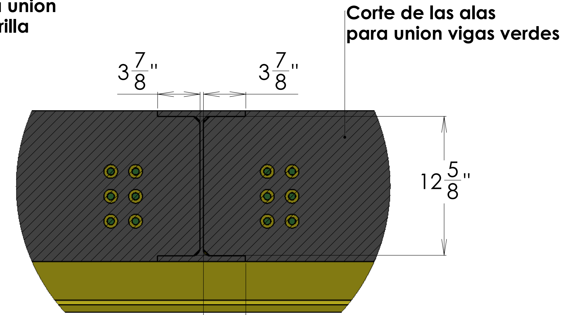
DETALLE K ESCALA 1:5
