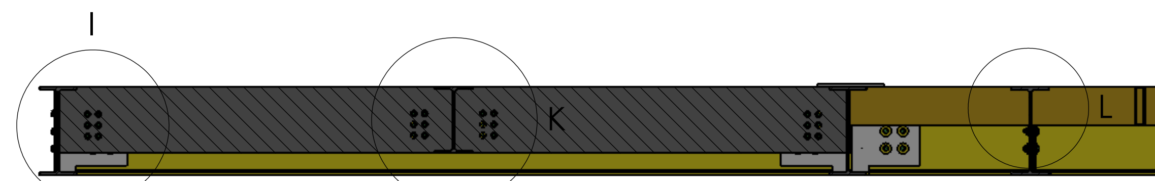
SECCIÓN H-H
